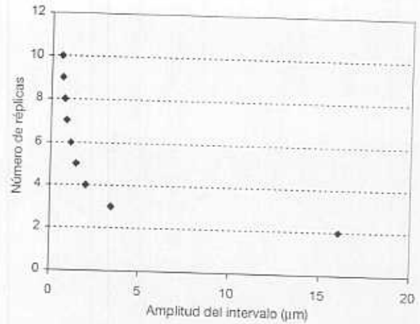
Figura 3. Variación de la amplitud del intervalo de confianza para la serie correspondiente a 3 meses de exposición en relación al número de réplicas.
