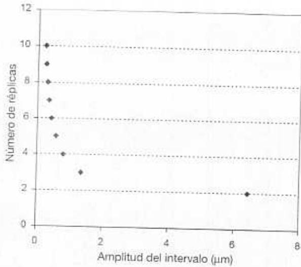
Figura 1. Variación de la amplitud del intervalo de confianza para la serie correspondiente a 1 mes de exposición en relación al número de réplicas.
