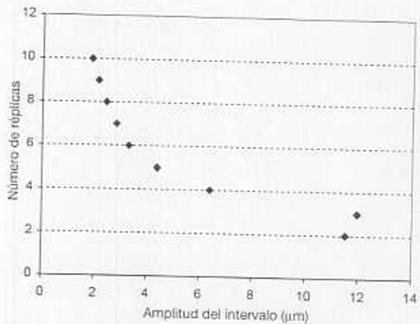
Figura 4. Variación de la amplitud del intervalo de confianza para la serie correspondiente a 7 meses de exposición en relación al número de réplicas.
